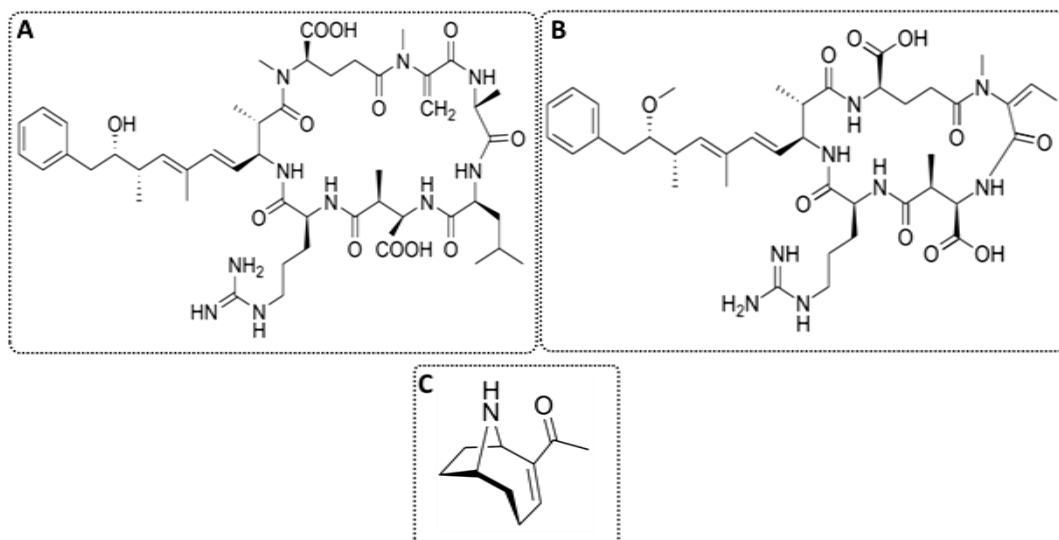
Figure 3 : Structures chimiques générales de la microcystine (A), la nodularine (B) et une neurotoxine (Anatoxine) (C) [6,10].
